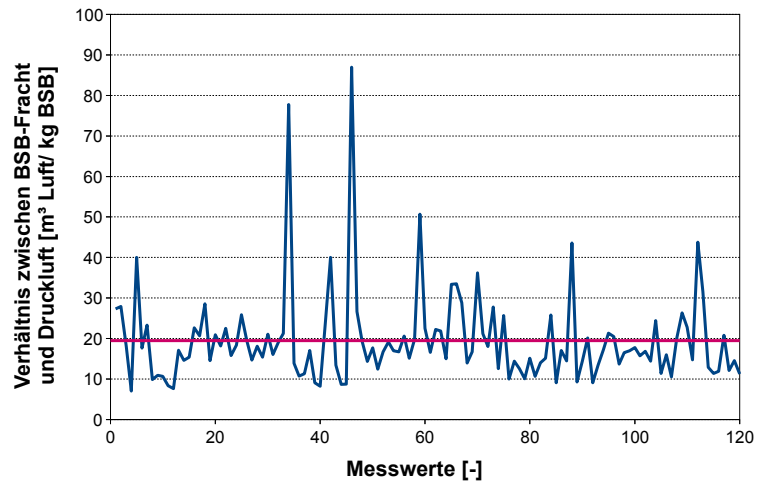
Bild 3 Spezifische Luftzufuhr pro kg BSB-Fracht
