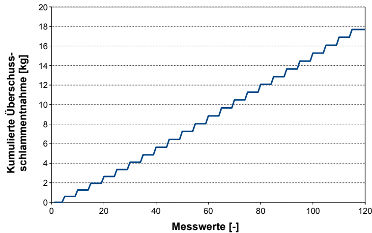
Bild 2 Kumulierte Überschussschlammmentnahmemenge über 120 Tage
